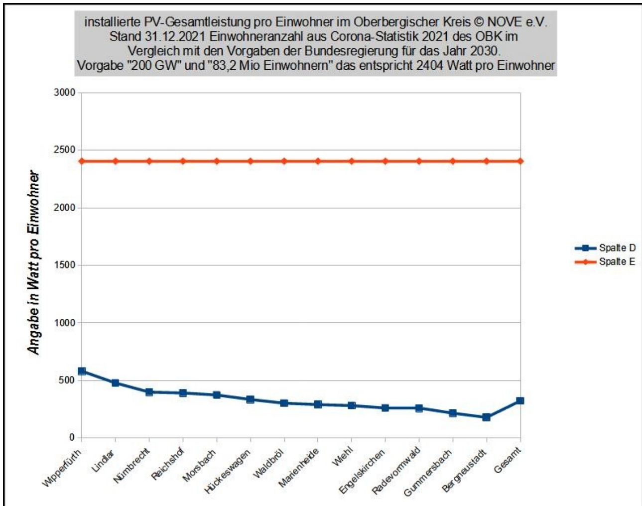
Bild 3. Installierte PV-Gesamtleistung im OBK pro Einwohner mit Zielvorgabe Stand 31.12.2021
