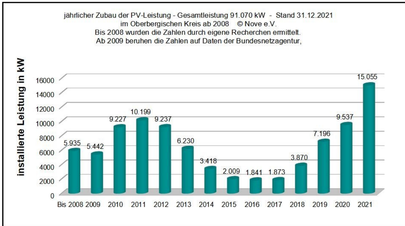
Bild 3. jährlicher Zubau ab 2008 bis 2021
